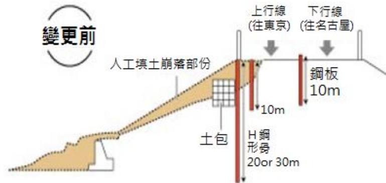
復原工程示意圖
