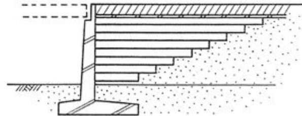
橋架背面填土(逆梯形)
